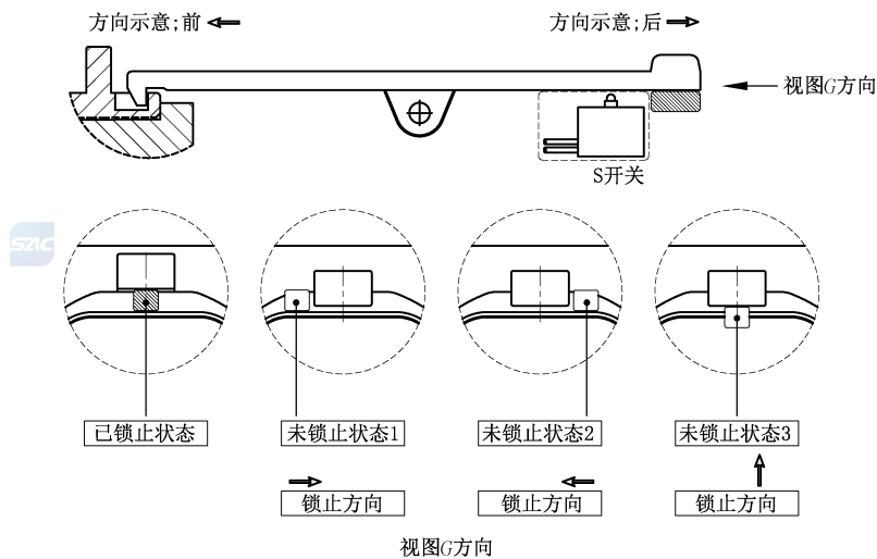
图 10 锁止装置结构示例 1
