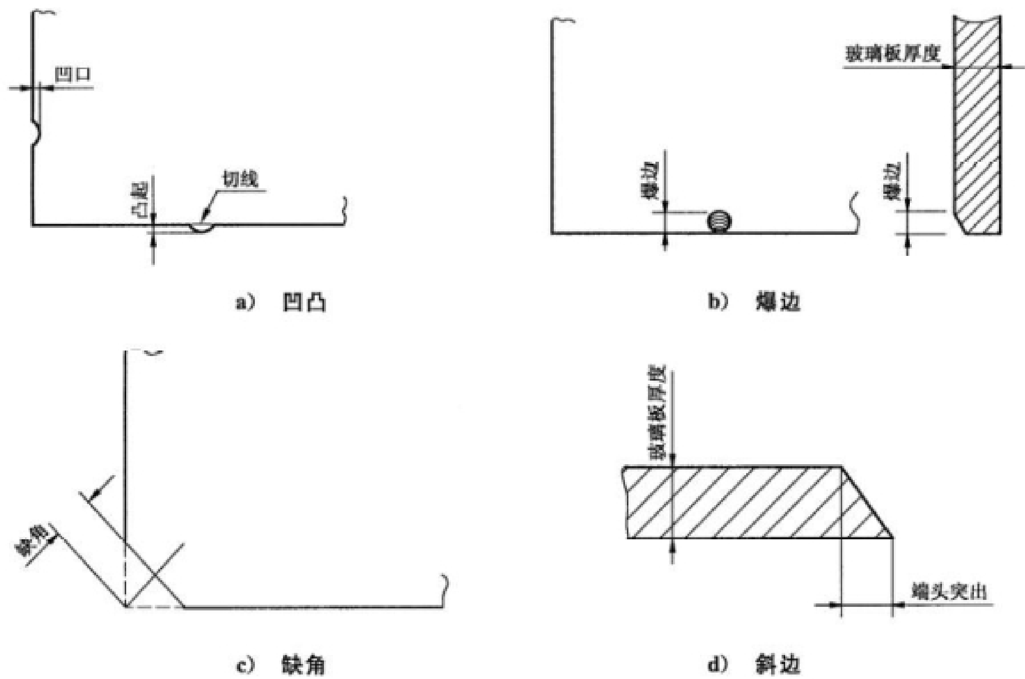
图 3 测量断面缺陷示意图
