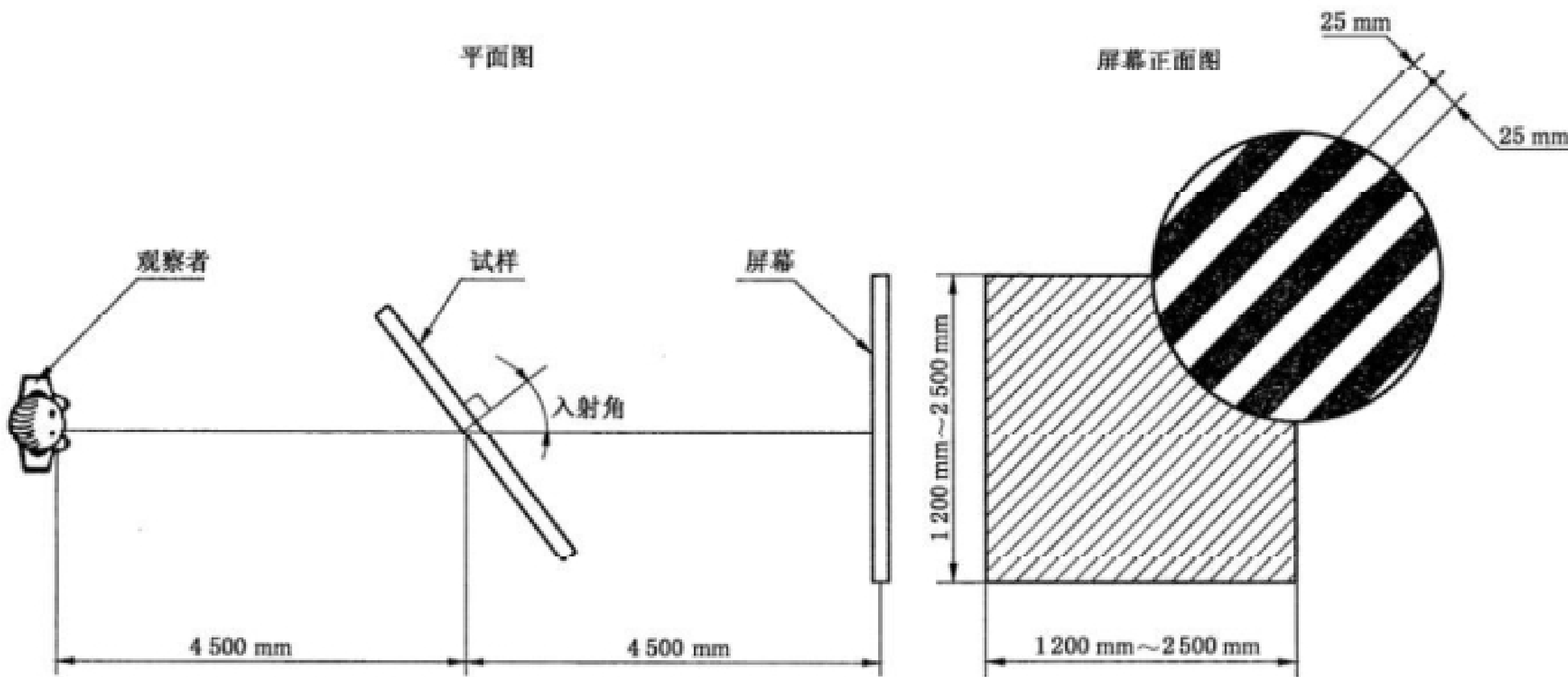
图 2 检验光学变形示意图
