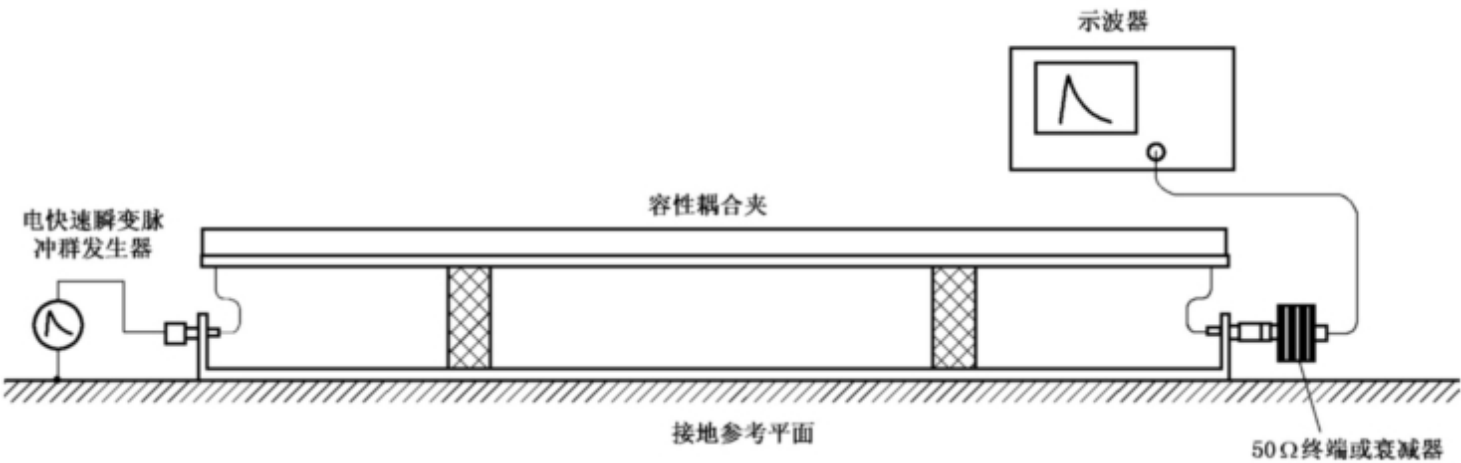
图 10 容性耦合夹验证布置示例
