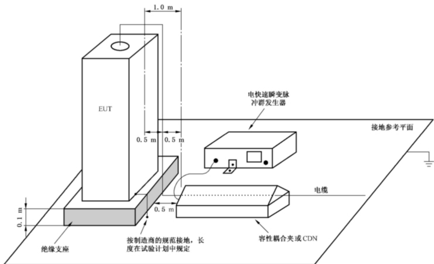
图 13 架高电缆的试验布置示例
