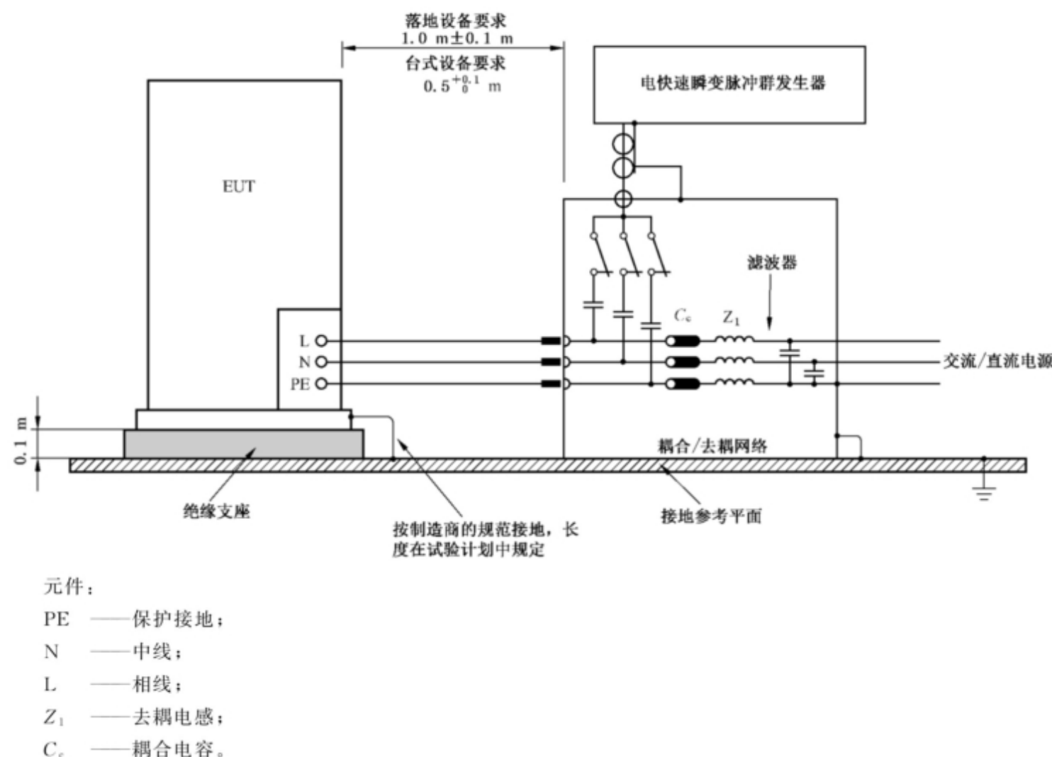
图 14 对交流/直流电源端直接耦合试验电压的实验室型式试验布置示例
