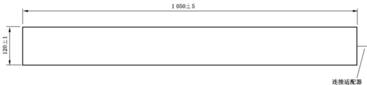
图 7 用于耦合夹校准的感应板
