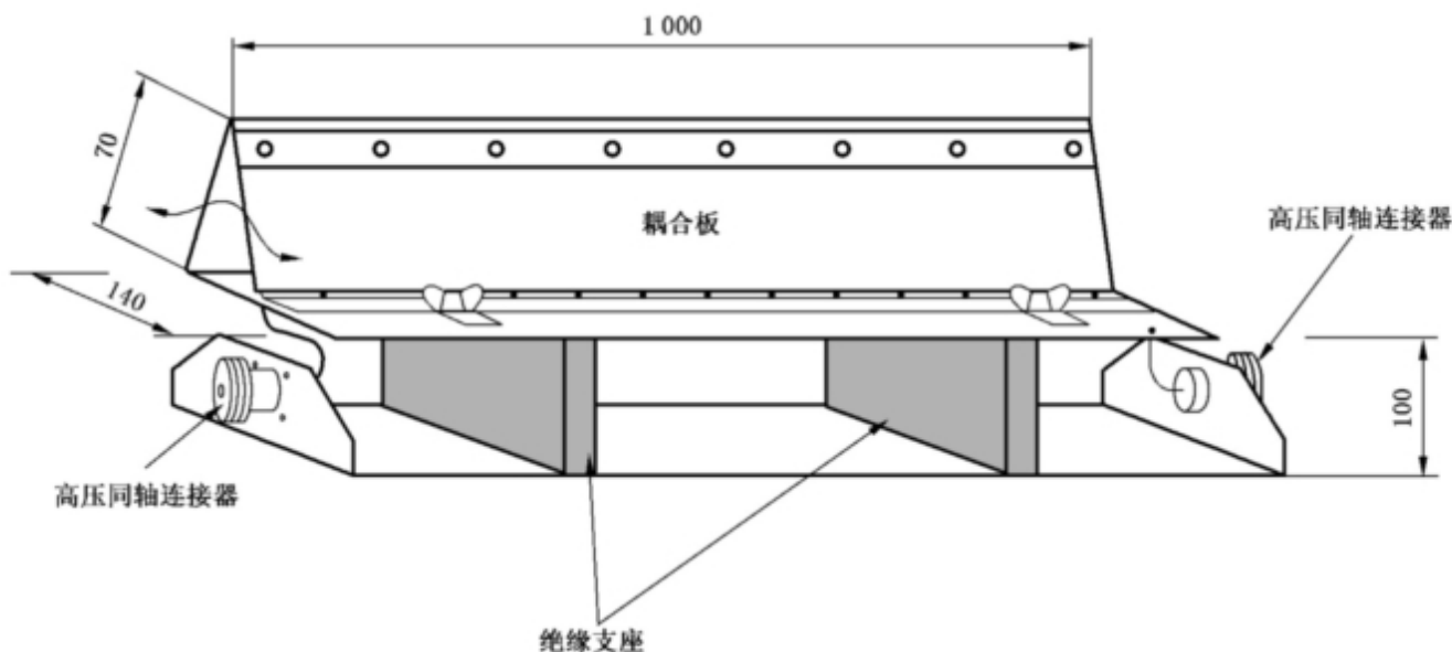
图 6 容性耦合夹结构
