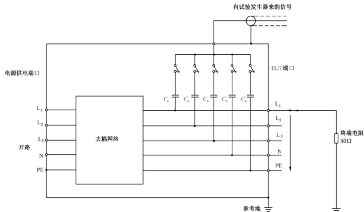
图 5 耦合/去耦网络输出端波形校准
