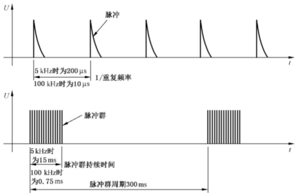
图 2 电快速瞬变脉冲群概略图
