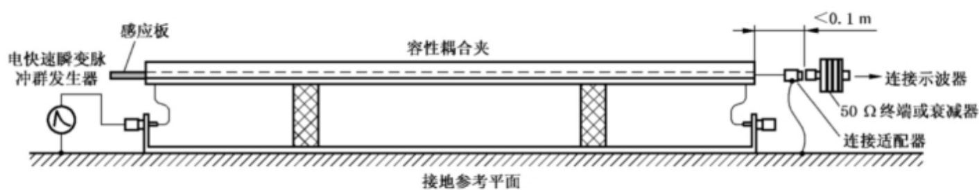
图 8 使用感应板校准容性耦合夹
