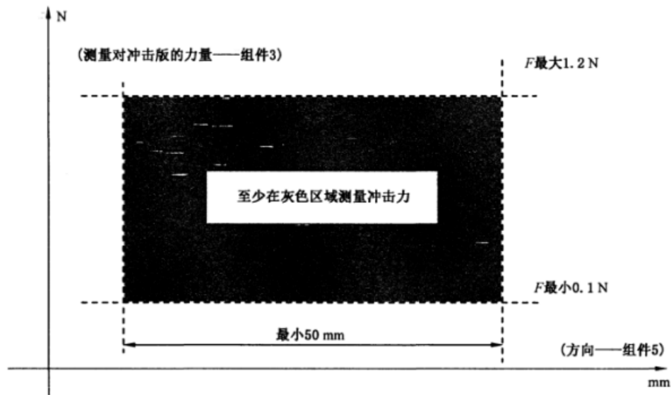
图 11 冲击力分布
