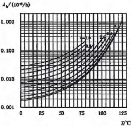
图 41 固体钽电解电容器基本失效率曲线
