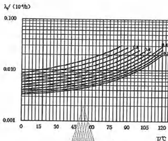
图 23 箔式电阻器基本失效率曲线
