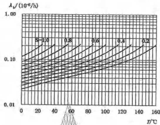
图 11 开关晶体管基本失效率曲线
