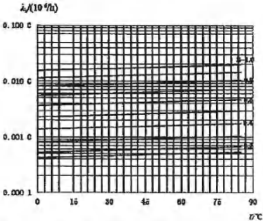
图 38 2 类瓷介电容器基本失效率曲线(额定温度为 85℃)
