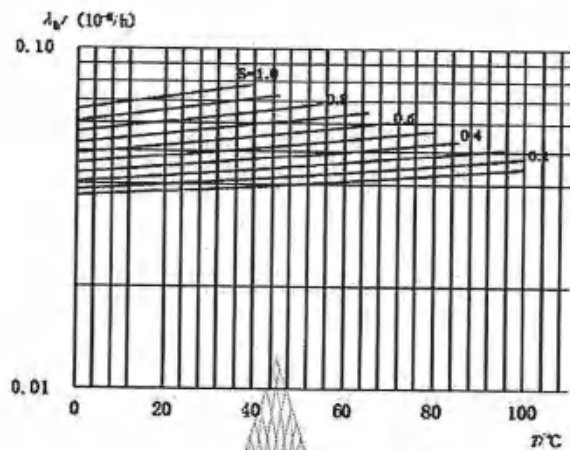
图 24 功率非线性电阻器基本失效率曲线
