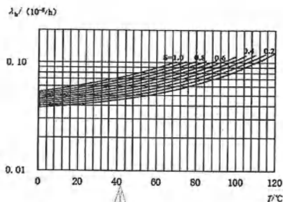
图 30 玻璃釉电位器基本失效率曲线
