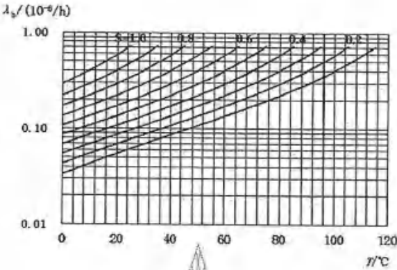
图 15 闸流晶体管基本失效率曲线
