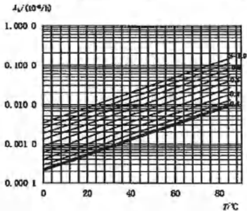
图 36 云母电容器基本失效率曲线(额定温度为 85℃)
