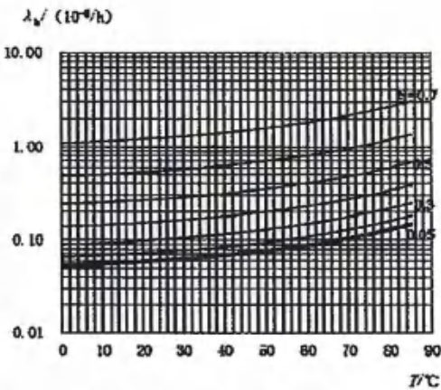
图 47 机电继电器感性负载基本失效率曲线(额定温度 85℃)
