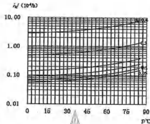
图 48 机电继电器灯负载基本失效率曲线(额定温度 85℃)
