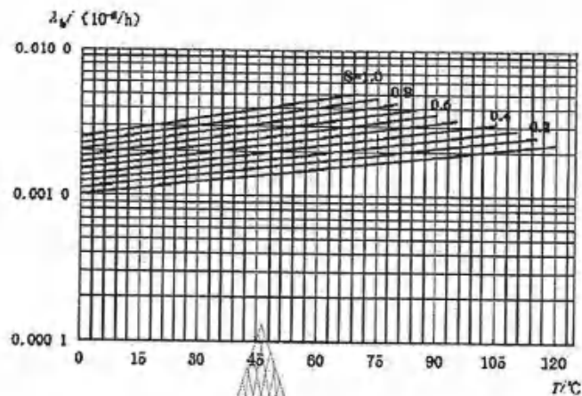
图 20 玻璃釉电阻器(功率 P \leq 2W ) 基本失效率曲线
