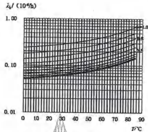
图 46 机电继电器阻性负载基本失效率曲线(额定温度 85℃)
