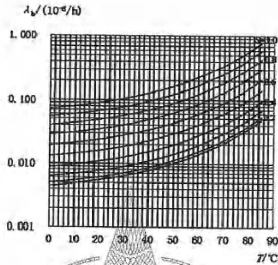
图 42 非固体钽电解电容器基本失效率曲线
