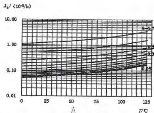
图 50 机电继电器感性负载基本失效率曲线(额定温度 125°C)
