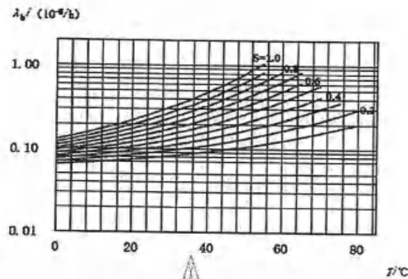
图 29 合成碳膜电位器基本失效率曲线
