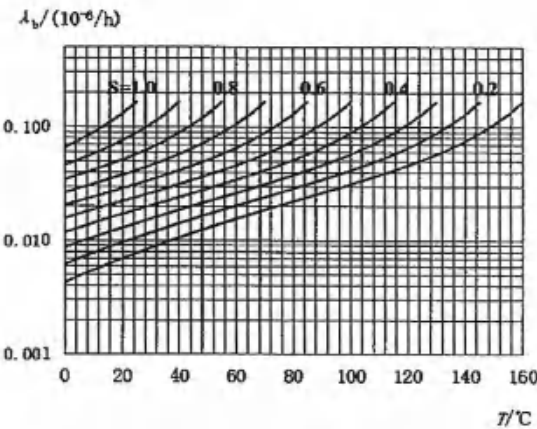
图 3 开关二极管基本失效率曲线
