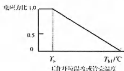
图 16 典型的降额曲线
