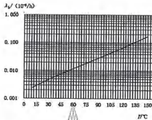
图 52 使用 I 类绝缘安装材料的低频连接器基本失效率曲线
