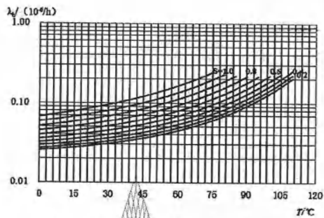
图 21 线绕电阻器基本失效率曲线
