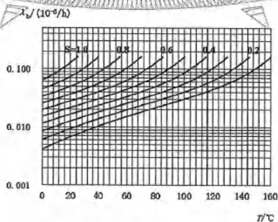
图 4 检波二极管基本失效率曲线
