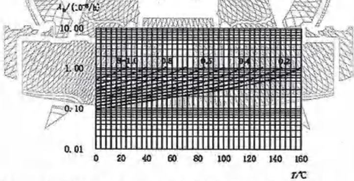
图 9 变容、阶跃、隧道、PIN、体效应与雪崩二极管基本失效率曲线
