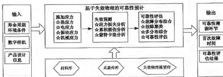
图 D.1 基于失效物理的可靠性预计一般流程
