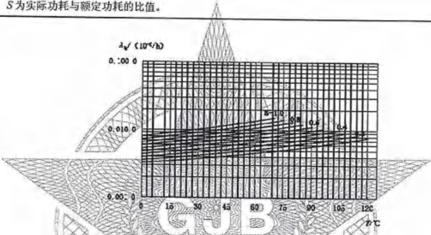
图 19 碳膜电阻器(功率 P \leq 2W ) 基本失效率曲线
