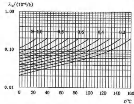
图 10 小功率晶体管和大功率晶体管基本失效率曲线
