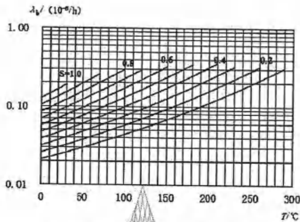
图 22 功率线绕电阻器基本失效率曲线
