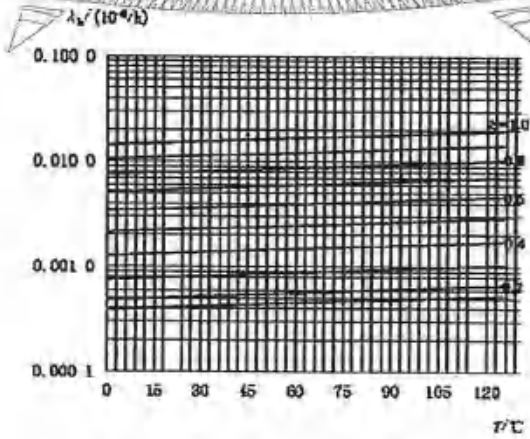
图 39 2 类瓷介电容器基本失效率曲线(额定温度为 125℃)
