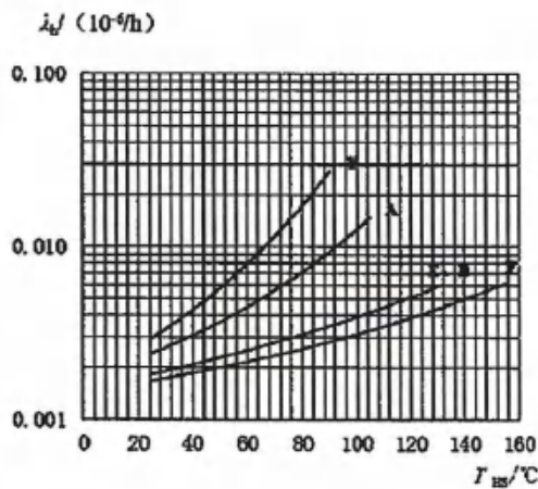
图 44 电感器基本失效率曲线
