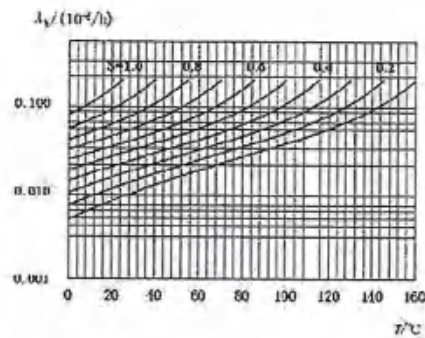
图 5 瞬态抑制二极管基本失效率曲线
