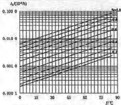
图 37 1 类瓷介电容器基本失效率曲线
