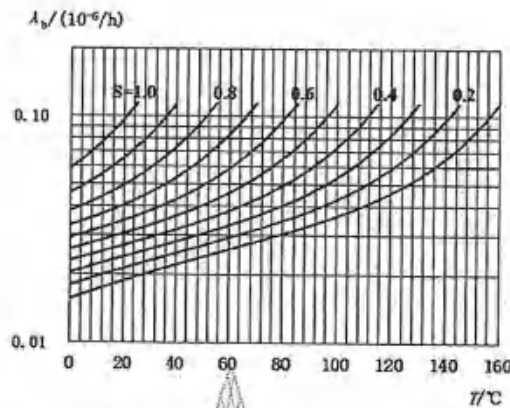
图 6 电压调整、电压基准及电流调整二极管基本失效率曲线
