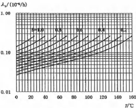
图 12 达林顿晶体管基本失效率曲线
