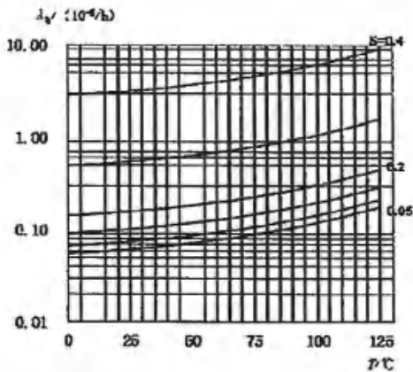
图 51 机电继电器灯负载基本失效率曲线(额定温度 125℃)
