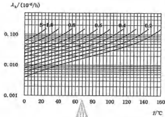
图 2 整流二极管基本失效率曲线
