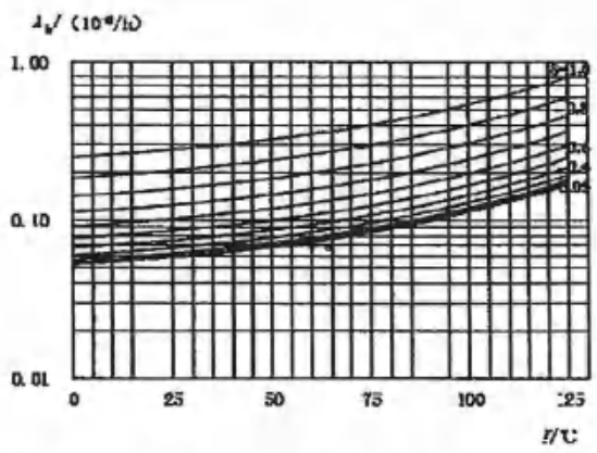
图 49 机电继电器阻性负载基本失效率曲线(额定温度 125℃)
