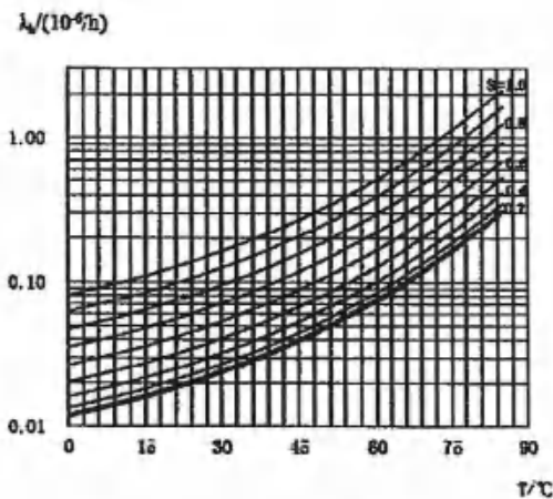
图 40 铝电解电容器基本失效率曲线
