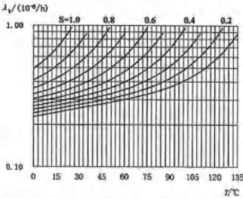
图 8 微波硅混频二极管基本失效率曲线
