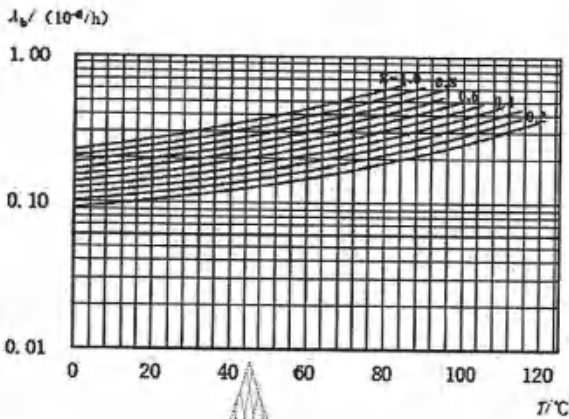
图 31 非线性精密电位器基本失效率曲线
