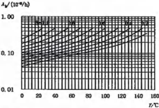
图 13 硅场效应晶体管基本失效率曲线
