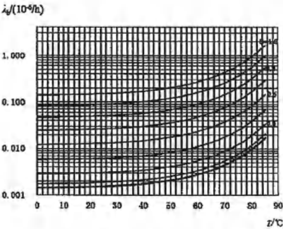
图 33 纸和薄膜电容器基本失效率曲线(额定温度为 85℃)
