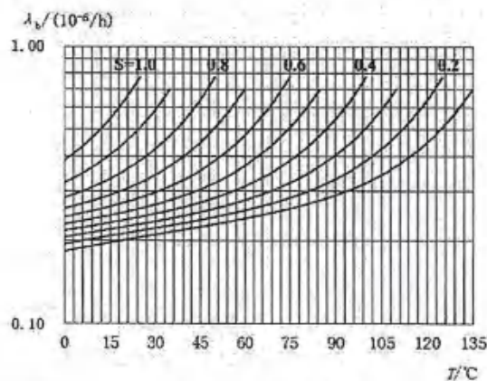
图 7 微波硅检波二极管基本失效率曲线
