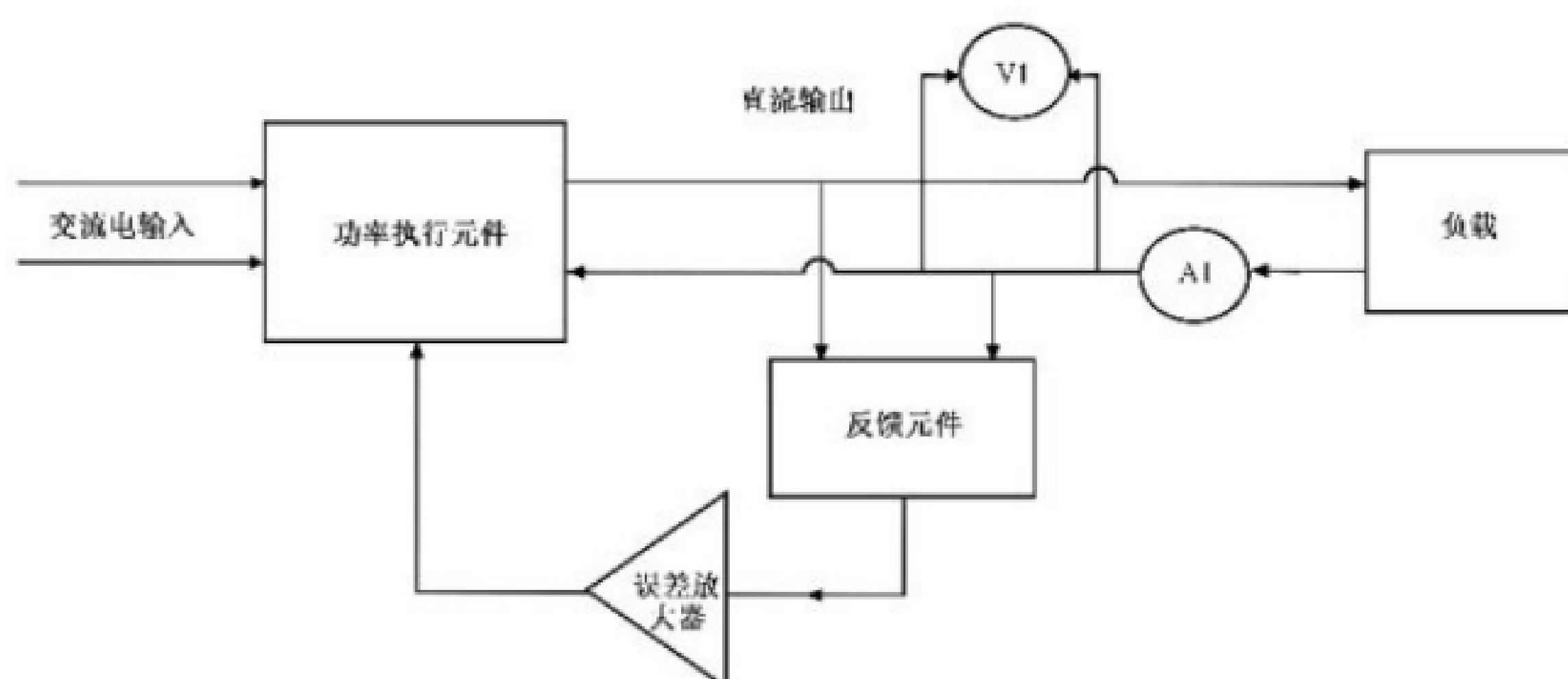
图 5 充电器元件失效测量原理框架
