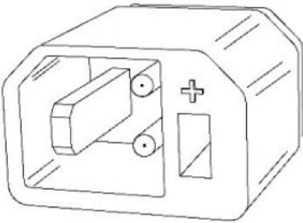
图 1 铅酸蓄电池充电器输出插头形式
