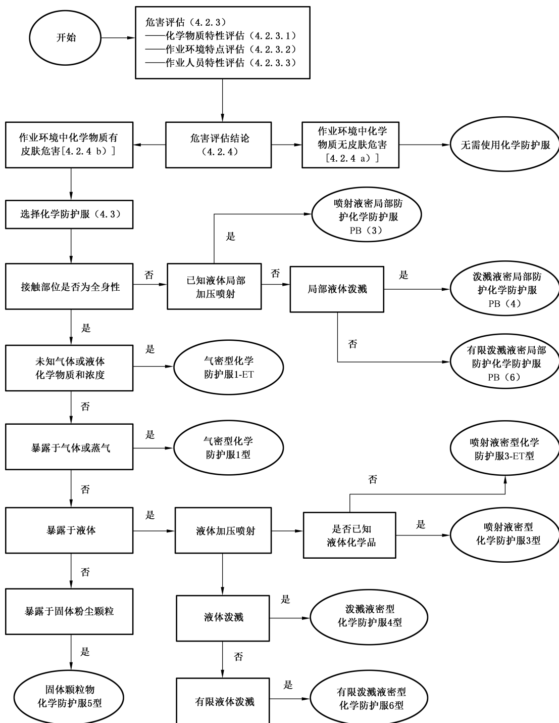
图 1 化学防护服的选择流程图
