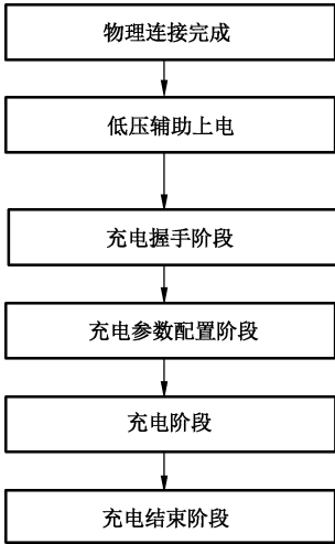
图 1 充电总体流程图
